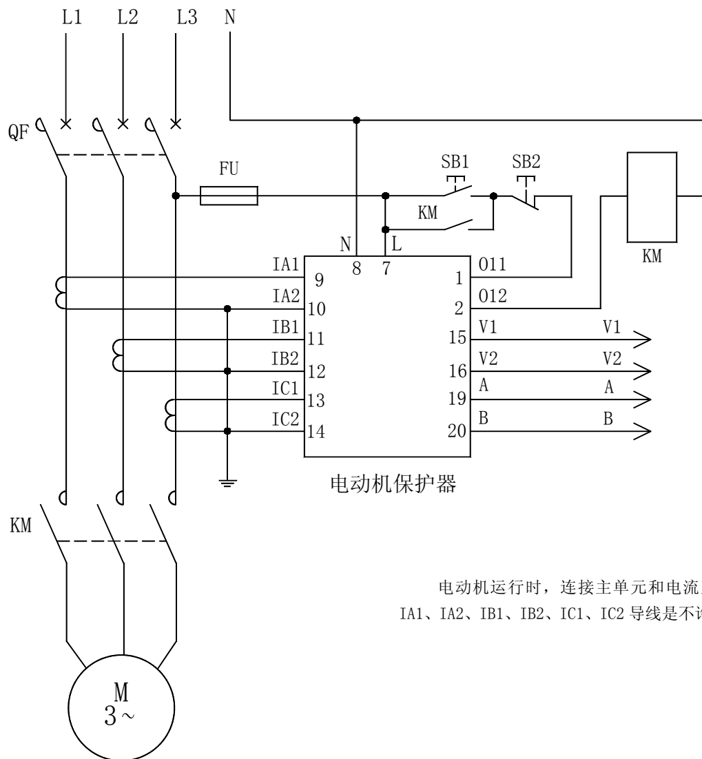
AMDP-X/F24□ 系列电动机保护器应用电气原理图
