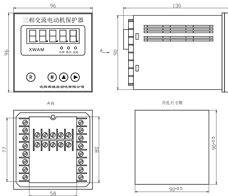
AMDP-X/F24□ 系列电动机保护器主单元外形及安装孔尺寸
