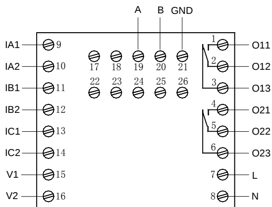
AMDP-X/F242 系列保护器主单元接线端子图
