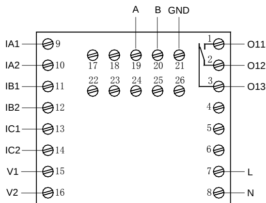
AMDP-X/F241 系列保护器主单元接线端子图
