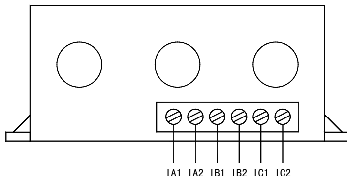
AMDPH-□/□C10□ 系列保护器电流检测单元接线端子图
