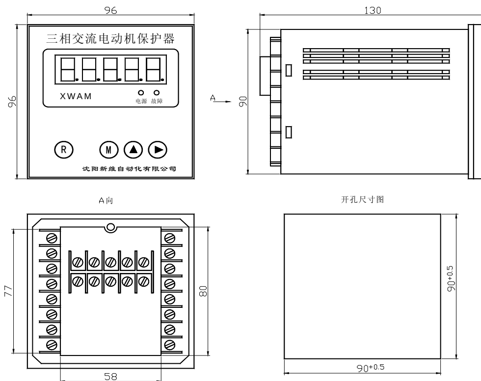
AMDPH-□/□C10□ 系列电动机保护器主单元外形及安装孔尺寸
