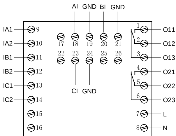
AMDPH-□/C102 系列保护器主单元接线端子图
