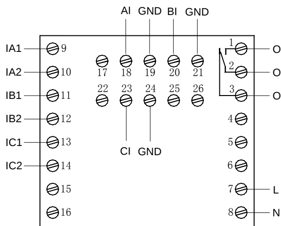
AMDPH-□/C101 系列保护器主单元接线端子图
