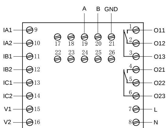
AMDPH-□/D232 系列保护器主单元接线端子图
