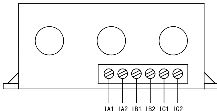
AMDPH-□/D23□ 系列保护器电流检测单元接线端子图
