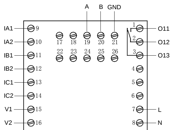
AMDPH-□/D231 系列保护器主单元接线端子图
