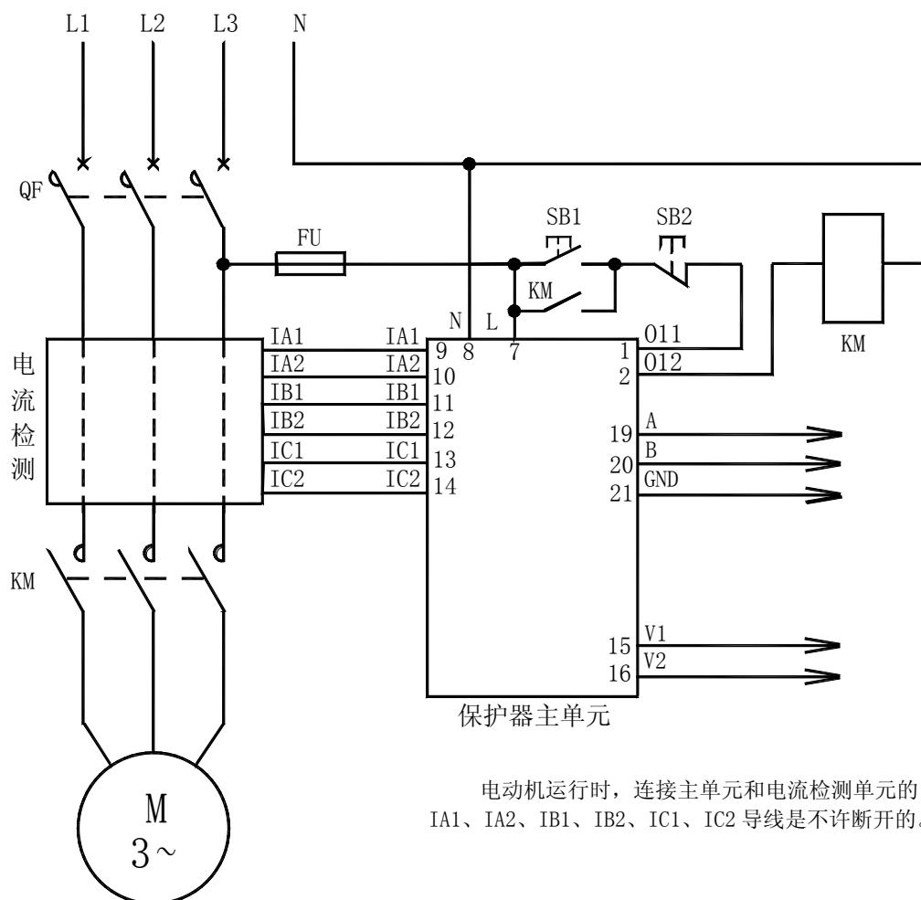
AMDPH-□/D23□ 系列电动机保护器应用电气原理图
