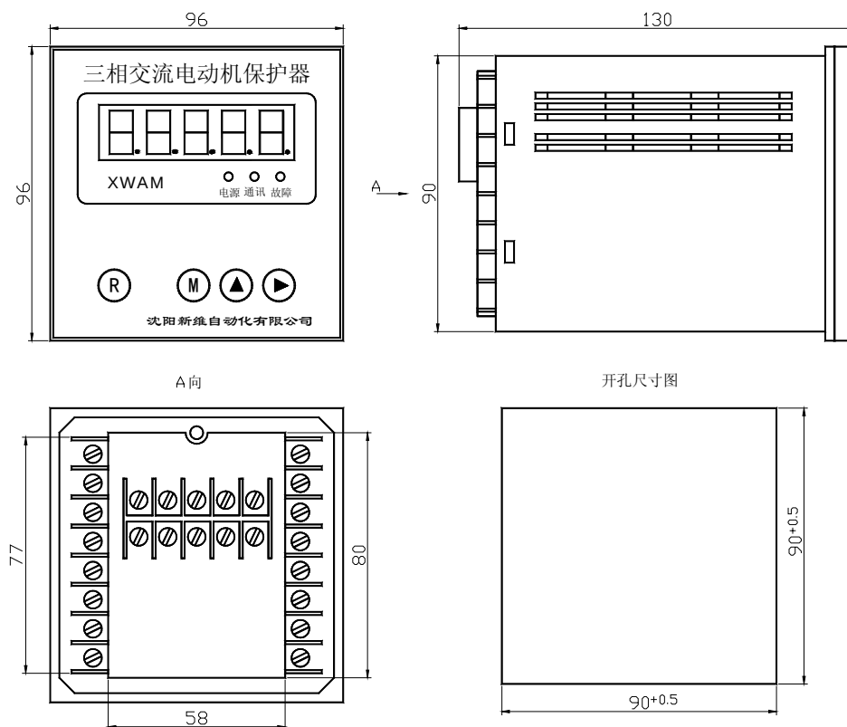
AMDPH-□/D23□ 系列电动机保护器主单元外形及安装孔尺寸
