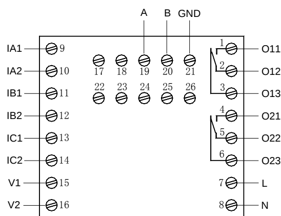
AMDPH-□/D332 系列保护器主单元接线端子图
