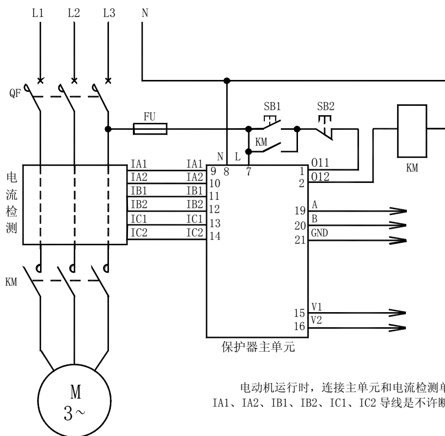
AMDPH-□/D33□ 系列电动机保护器应用电气原理图
