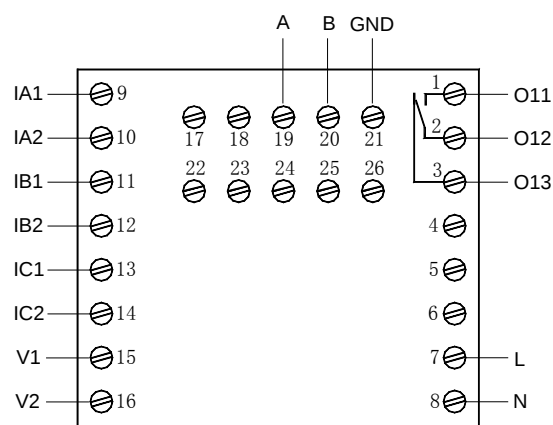
AMDPH-□/D331 系列保护器主单元接线端子图
