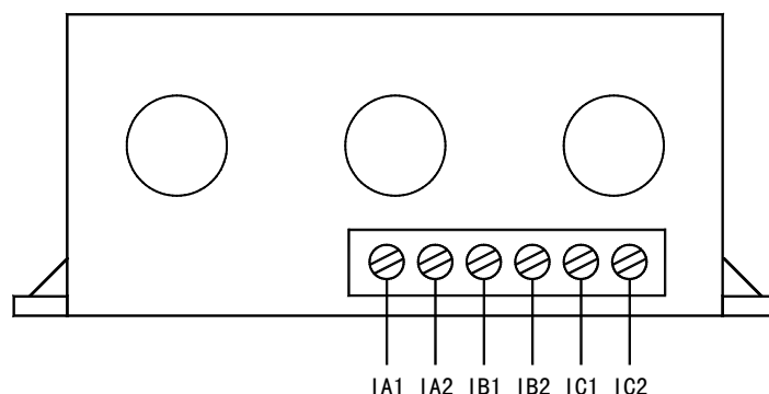
AMDPH-□/D33□ 系列保护器电流检测单元接线端子图
