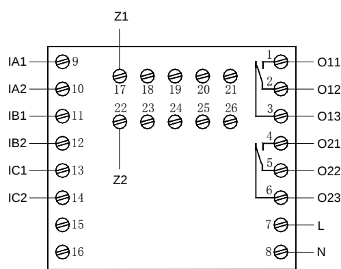
AMDPH-X/E012 系列保护器主单元接线端子图
