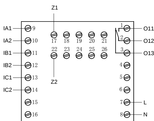
AMDPH-X/E011 系列保护器主单元接线端子图
