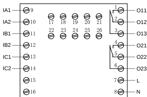
AMDPH-X/E022 系列保护器主单元接线端子图 HTTP://WWW.SY-XINWEI.COM
