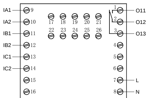
AMDPH-X/E021 系列保护器主单元接线端子图 沈阳新维自动化有限公司
