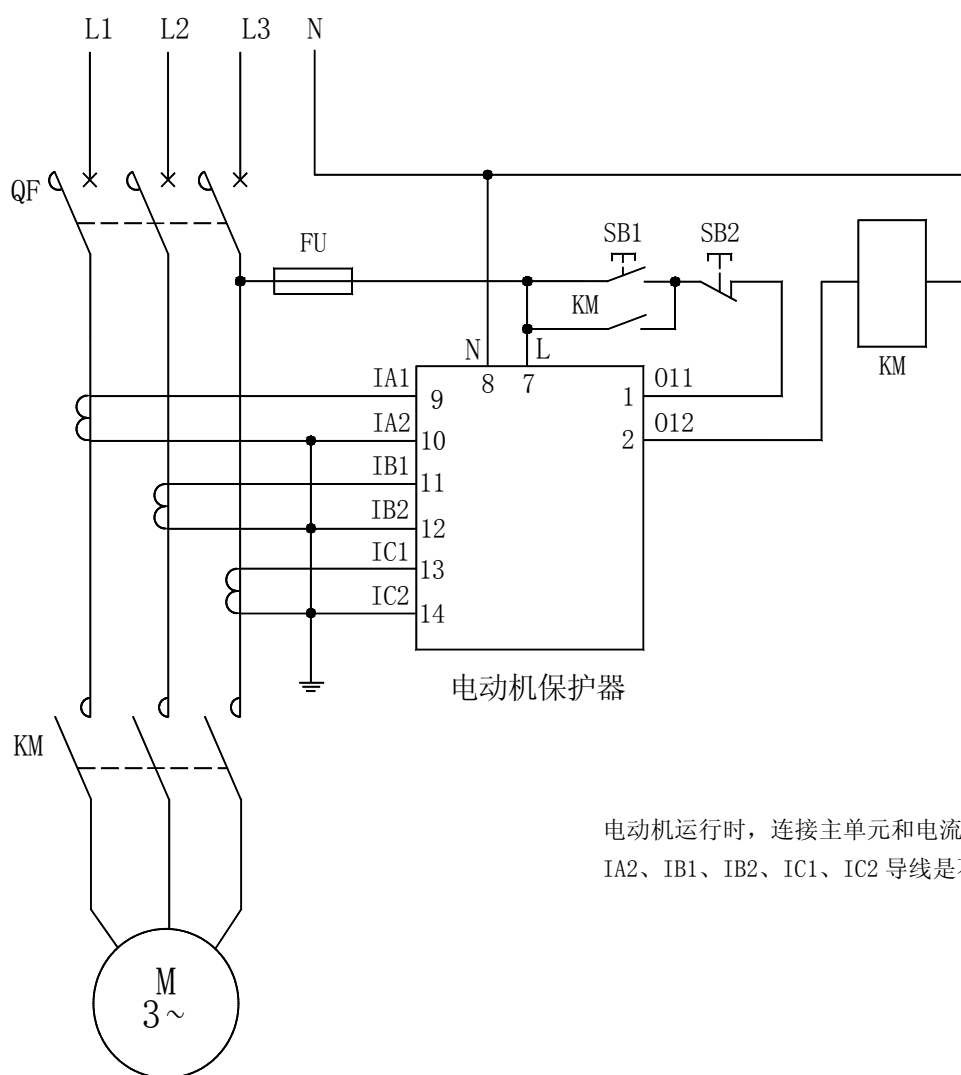
AMDPH-X/E02□ 系列电动机保护器应用电气原理图
