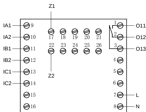
AMDPH-X/E051 系列保护器主单元接线端子图
