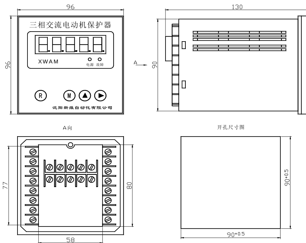
AMDPH-X/E05□ 系列电动机保护器主单元外形及安装孔尺寸
