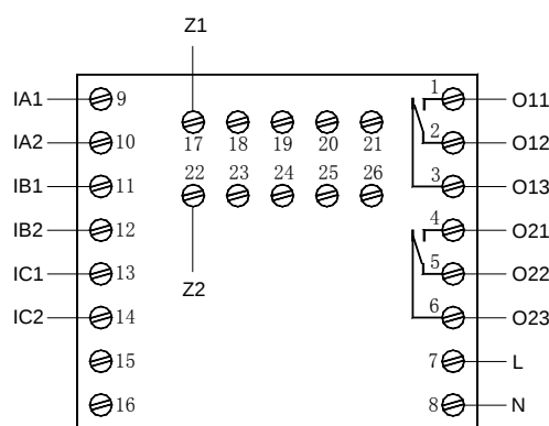
AMDPH-X/E052 系列保护器主单元接线端子图
