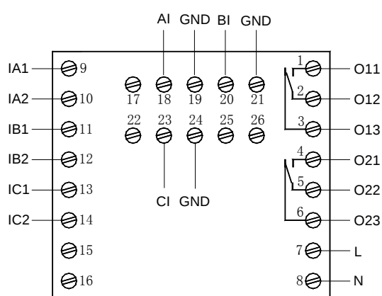
AMDPH-X/E102 系列保护器主单元接线端子图
