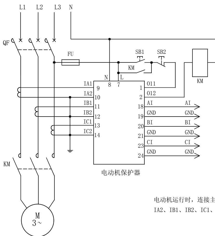
AMDPH-X/E10□ 系列电动机保护器应用电气原理图
