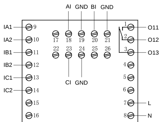
AMDPH-X/E101 系列保护器主单元接线端子图
