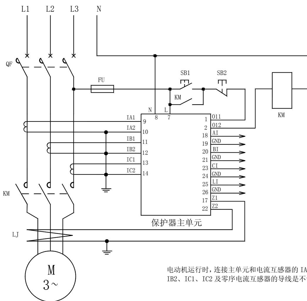
AMDPH-X/E11□ 系列电动机保护器应用电气原理图
