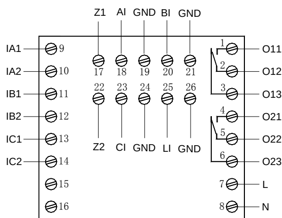
AMDPH-X/E112 系列保护器主单元接线端子图
