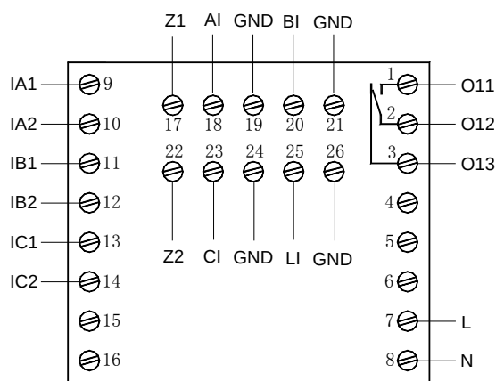
AMDPH-X/E111 系列保护器主单元接线端子图
