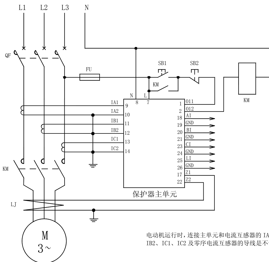
AMDPH-X/E15□ 系列电动机保护器应用电气原理图
