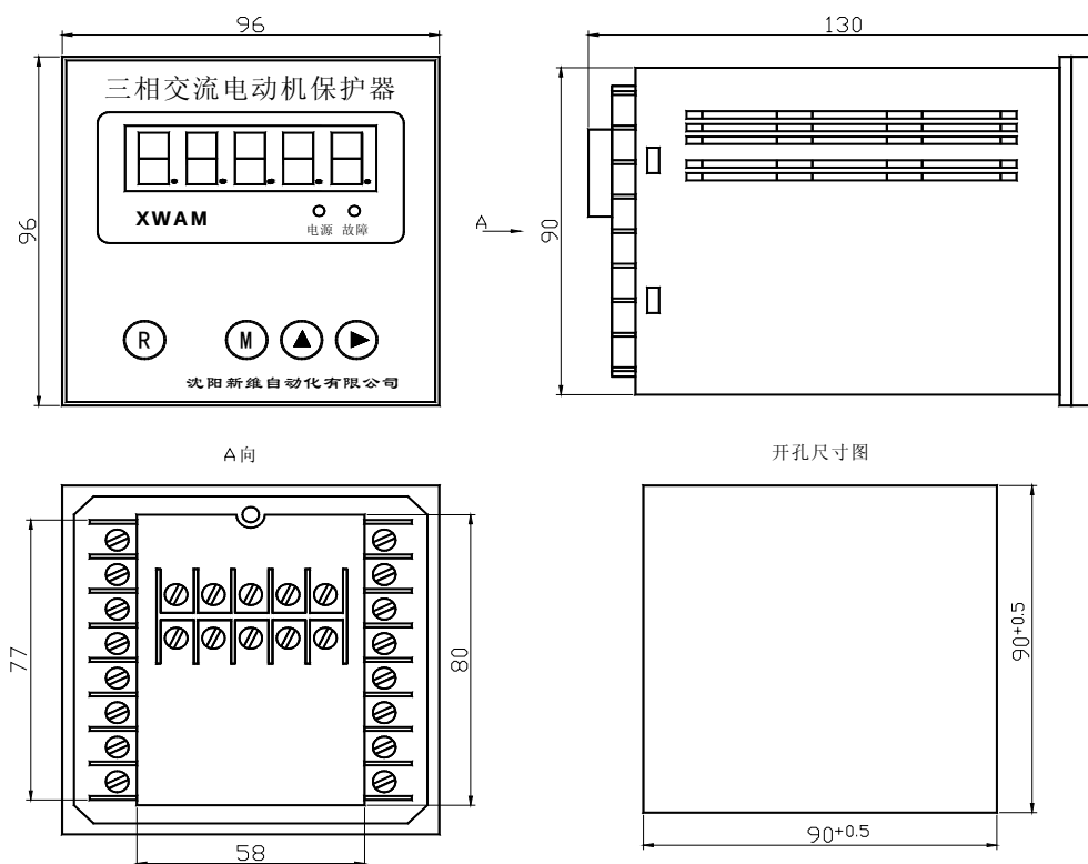
AMDPH-X/E15□ 系列电动机保护器主单元外形及安装孔尺寸
