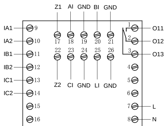
AMDPH-X/E151 系列保护器主单元接线端子图
