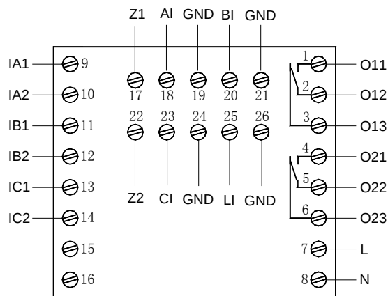
AMDPH-X/E152 系列保护器主单元接线端子图
