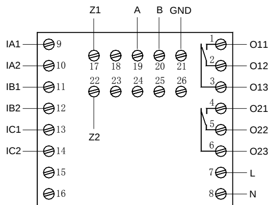
AMDPH-X/E252 系列保护器主单元接线端子图
