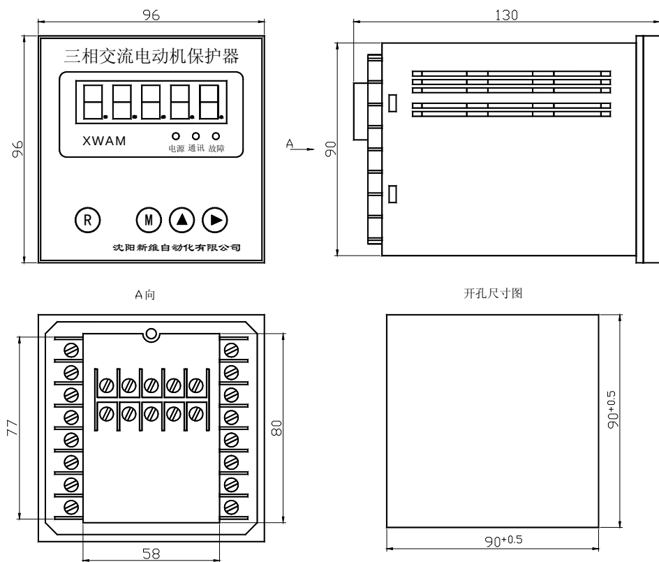
AMDPH-X/E25□ 系列电动机保护器主单元外形及安装孔尺寸
