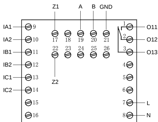
AMDPH-X/E251 系列保护器主单元接线端子图
