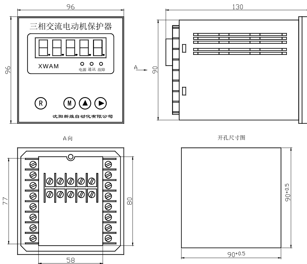
AMDPH-X/E30□ 系列电动机保护器主单元外形及安装孔尺寸
