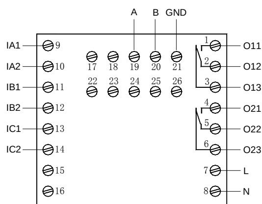
AMDPH-X/E302 系列保护器主单元接线端子图
