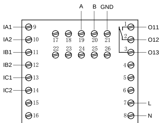
AMDPH-X/E301 系列保护器主单元接线端子图
