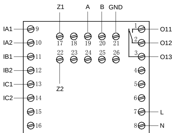
AMDPH-X/E311 系列保护器主单元接线端子图
