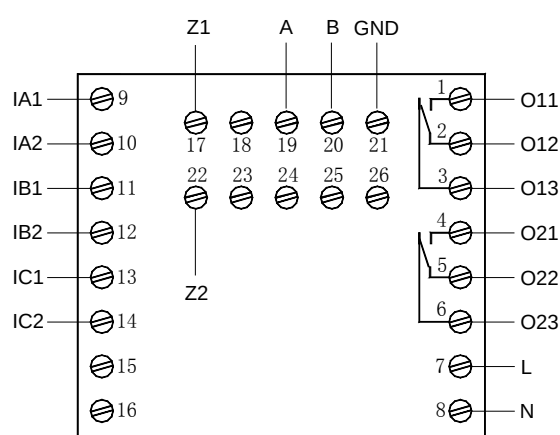
AMDPH-X/E312 系列保护器主单元接线端子图
