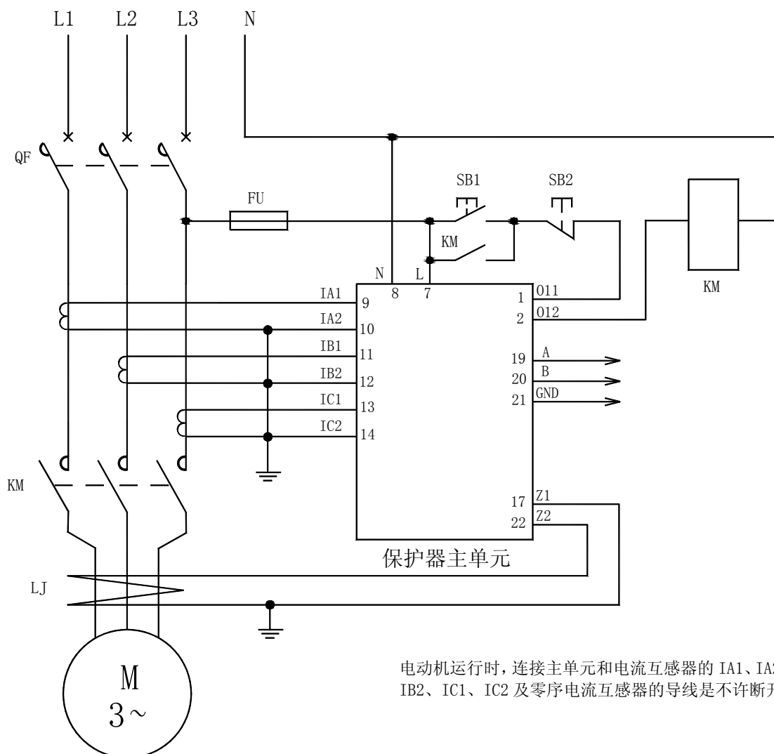
AMDPH-X/E31□ 系列电动机保护器应用电气原理图
