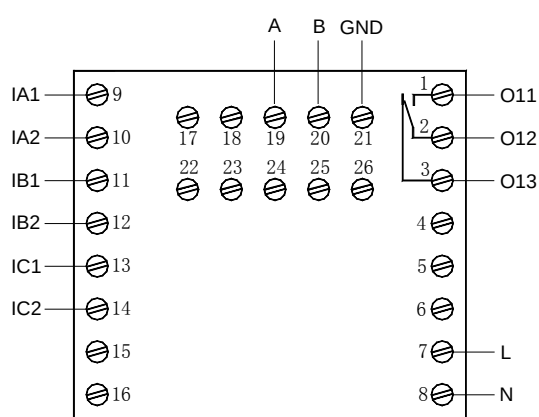
AMDPH-X/E321 系列保护器主单元接线端子图
