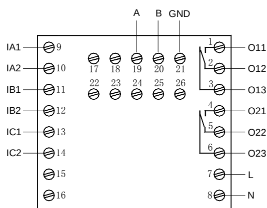
AMDPH-X/E322 系列保护器主单元接线端子图
