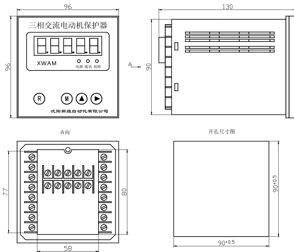
AMDPH-X/E32□ 系列电动机保护器主单元外形及安装孔尺寸
