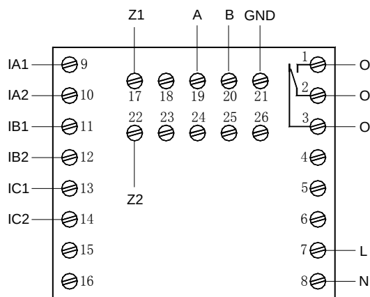
AMDPH-X/E351 系列保护器主单元接线端子图
