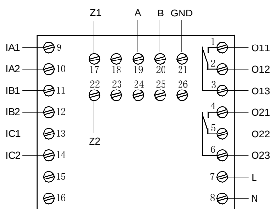
AMDPH-X/E352 系列保护器主单元接线端子图
