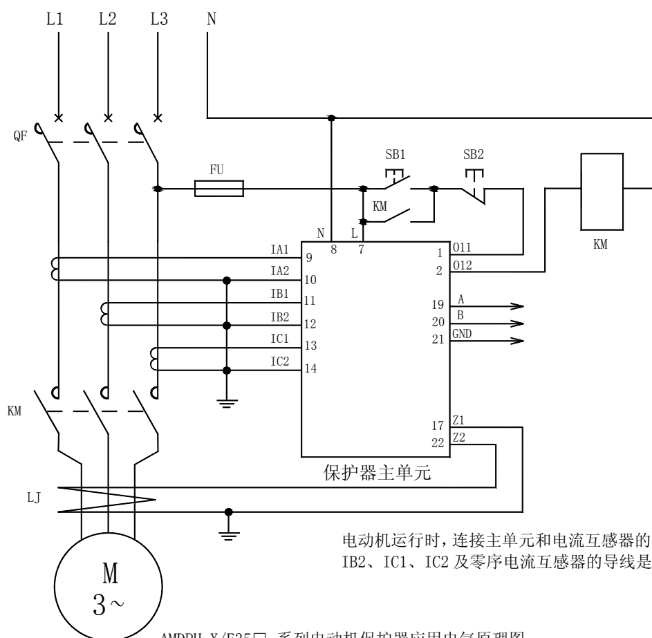
AMDPH-X/E351 系列电动机保护器应用电气原理图
