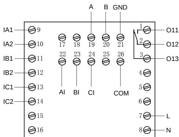
AMDPH-X/E401 系列保护器主单元接线端子图
