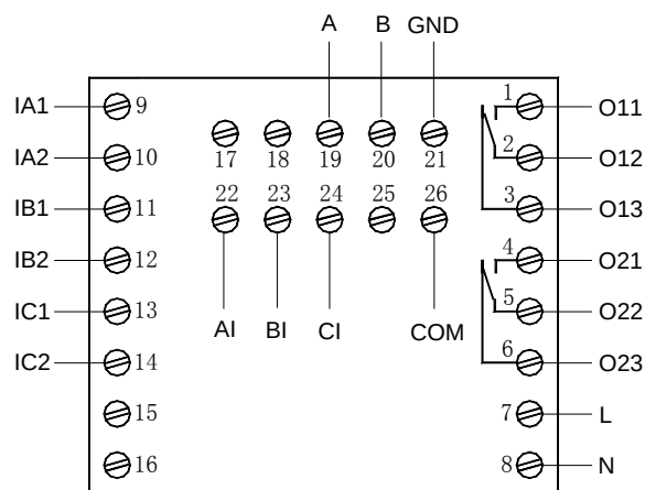
AMDPH-X/E402 系列保护器主单元接线端子图
