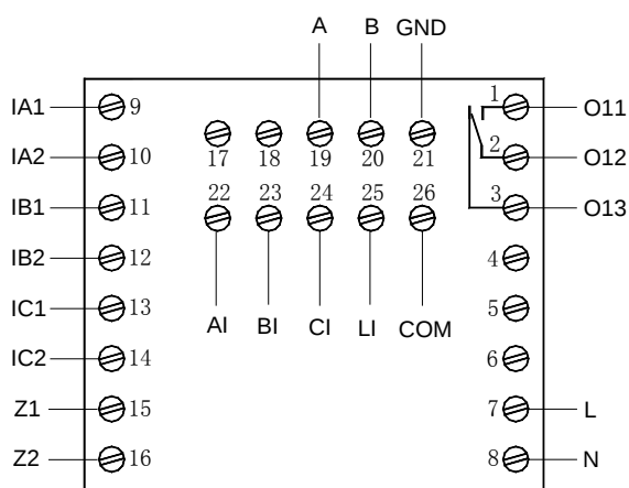
AMDPH-X/E411 系列保护器主单元接线端子图
