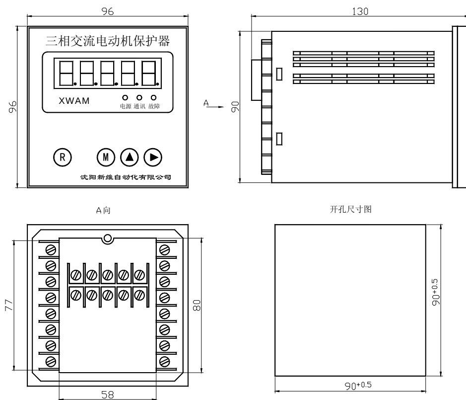
AMDPH-X/E41□ 系列电动机保护器主单元外形及安装孔尺寸
