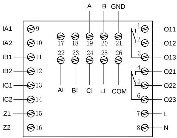
AMDPH-X/E412 系列保护器主单元接线端子图
