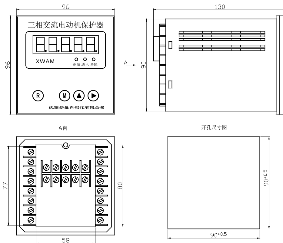
AMDPH-X/E42□ 系列电动机保护器主单元外形及安装孔尺寸
