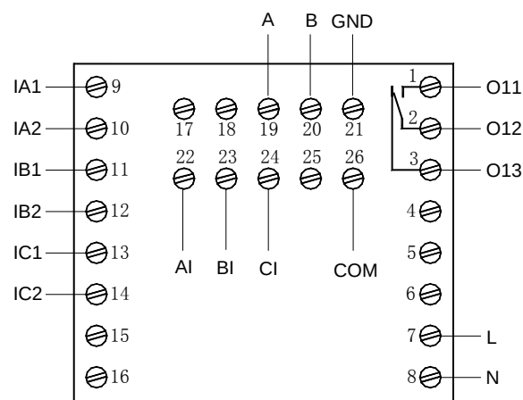
AMDPH-X/E421 系列保护器主单元接线端子图
