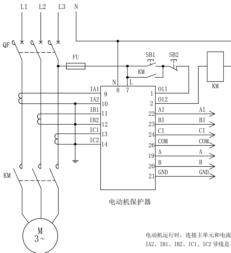
AMDPH-X/E42□ 系列电动机保护器应用电气原理图
