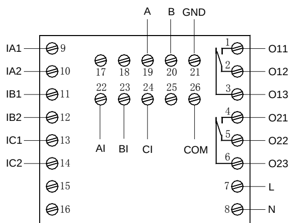
AMDPH-X/E422 系列保护器主单元接线端子图
