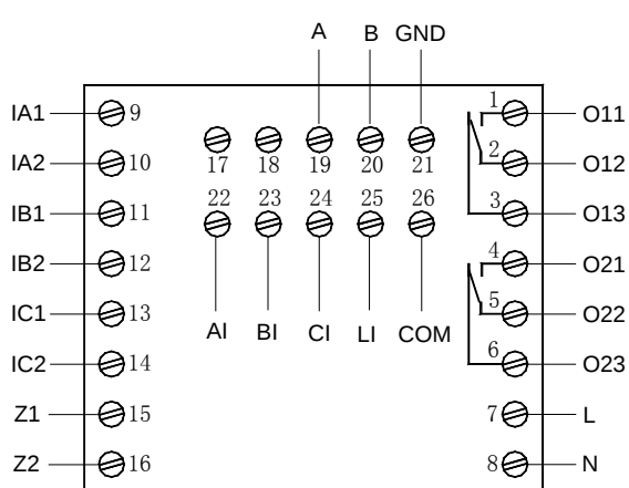
AMDPH-X/E452 系列保护器主单元接线端子图
