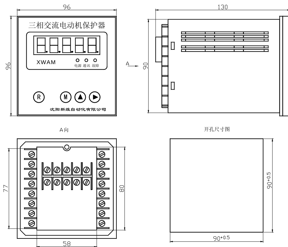
AMDPH-X/E45□ 系列电动机保护器主单元外形及安装孔尺寸
