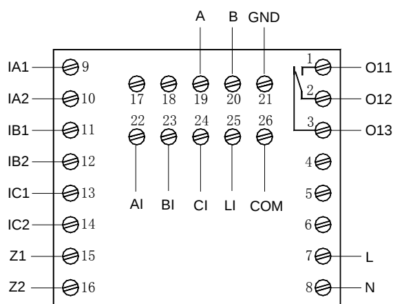
AMDPH-X/E451 系列保护器主单元接线端子图
