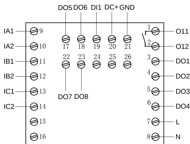
AMDPH-X/E501 系列保护器主单元接线端子图
