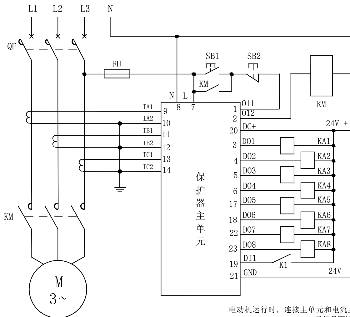
AMDPH-X/E501 系列电动机保护器 D0 连接继电器电气原理图
