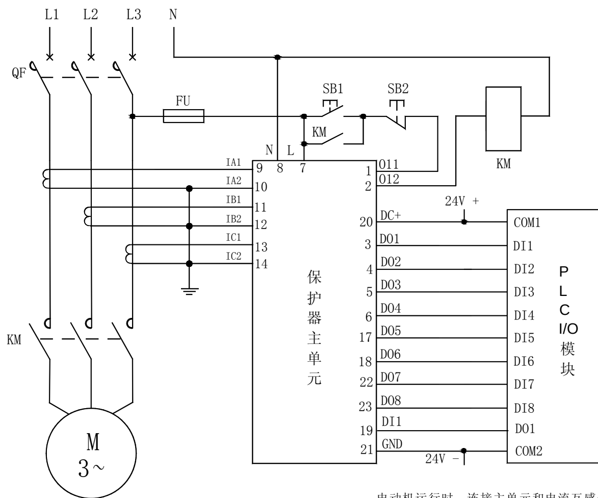
AMDPH-X/E501 系列电动机保护器 DO 连接 PLC 电气原理图
