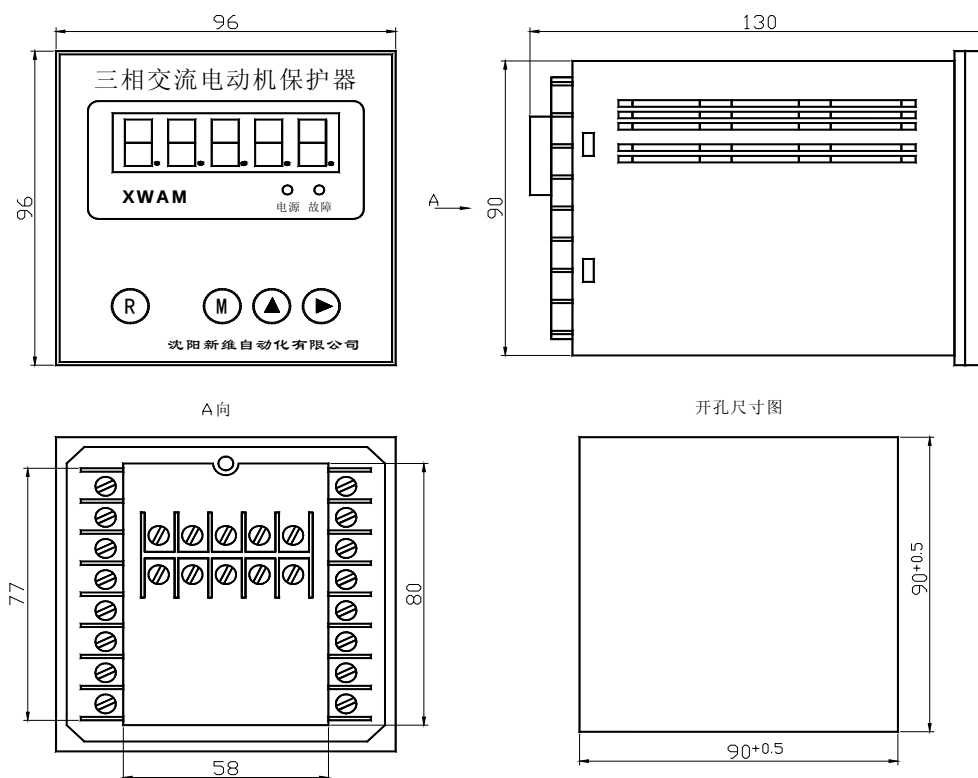
AMDPH-X/E511 系列电动机保护器主单元外形及安装孔尺寸
