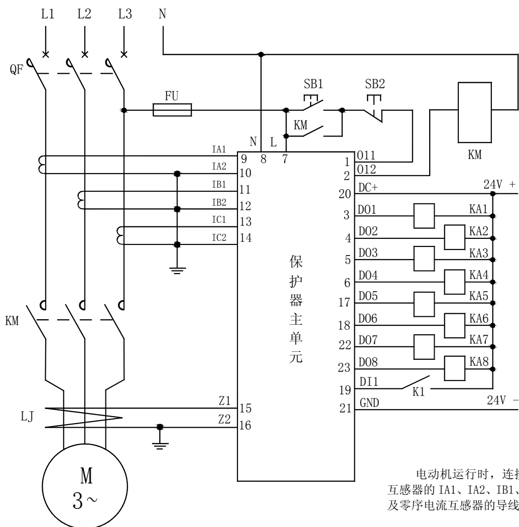
AMDPH-X/E511 系列电动机保护器 D0 连接继电器电气原理图
