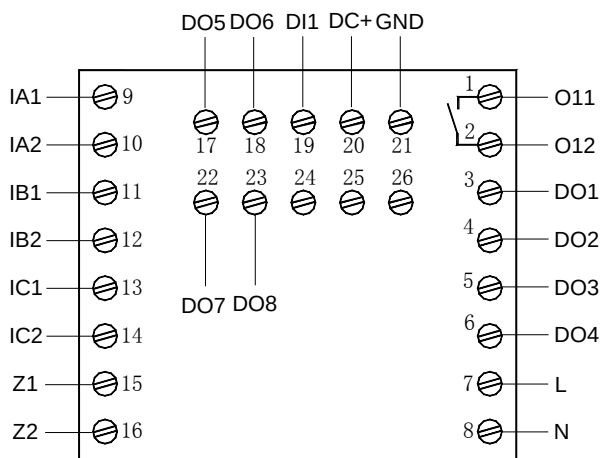
AMDPH-X/E511 系列保护器主单元接线端子图
