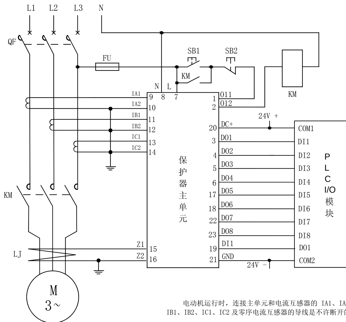
AMDPH-X/E511 系列电动机保护器 D0 连接 PLC 电气原理图
