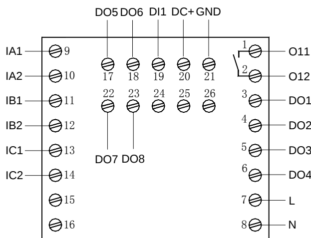
AMDPH-X/E521 系列保护器主单元接线端子图
