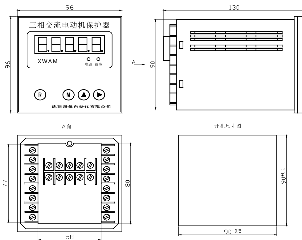
AMDPH-X/E521 系列电动机保护器主单元外形及安装孔尺寸
