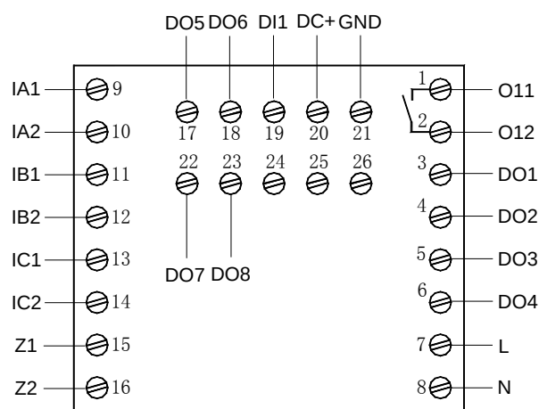
AMDPH-X/E551 系列保护器主单元接线端子图
