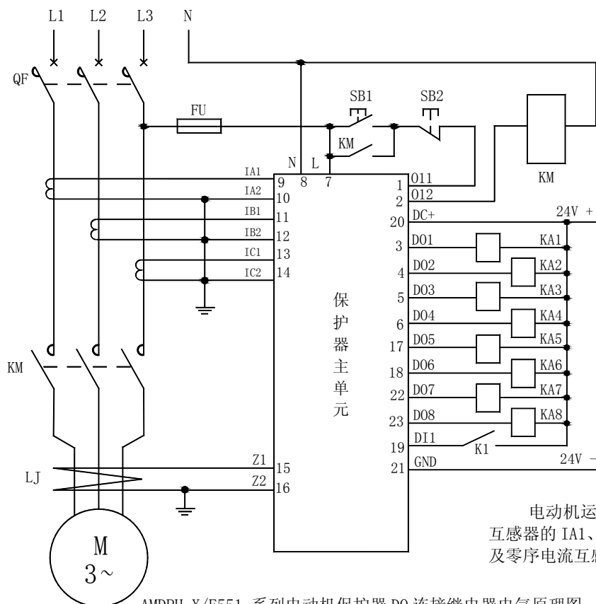
AMDPH-X/E551 系列电动机保护器 DO 连接继电器电气原理图
