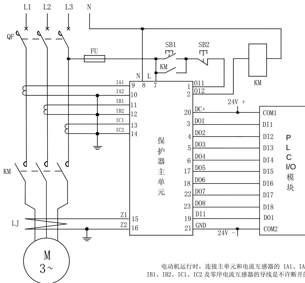
AMDPH-X/E551 系列电动机保护器 D0 连接 PLC 电气原理图
