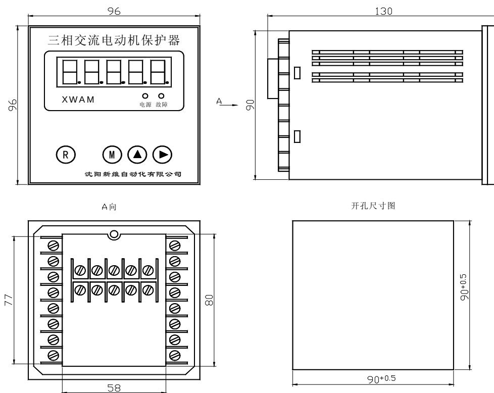
AMDPH-X/E551 系列电动机保护器主单元外形及安装孔尺寸
