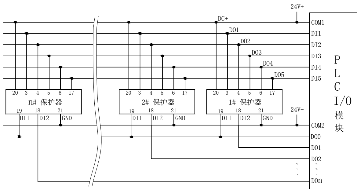
PLC 读取多台 AMDPH-X/E601 系列电动机保护器电气原理图
