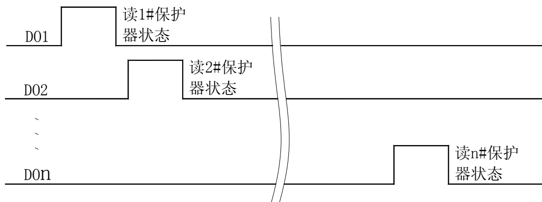
PLC 读取多台 AMDPH-X/E601 系列电动机保护器时序图
