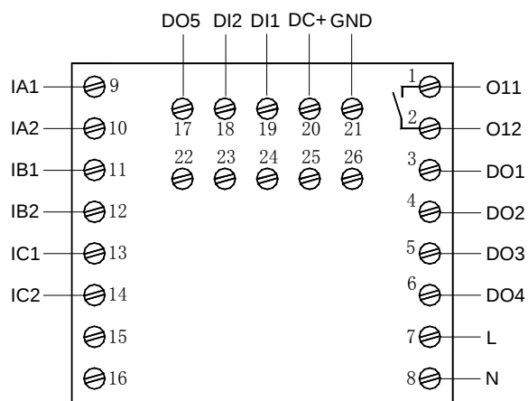
AMDPH-X/E601 系列保护器主单元接线端子图
