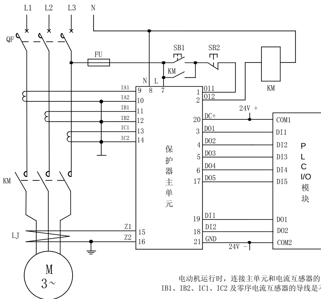
AMDP-X/E611 系列电动机保护器 DO 连接 PLC 电气原理图
