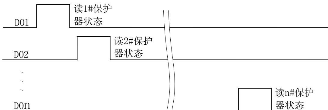
PLC 读取多台 AMDPH-X/E621 系列电动机保护器时序图
