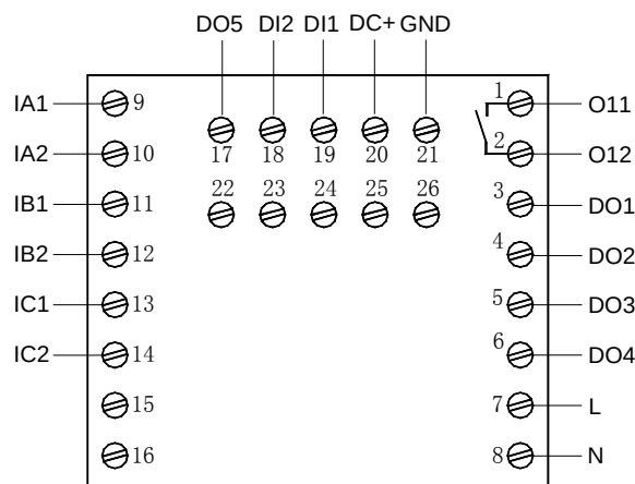
AMDPH-X/E621 系列保护器主单元接线端子图
