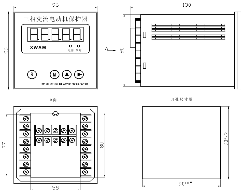
AMDPH-X/E621 系列电动机保护器主单元外形及安装孔尺寸
