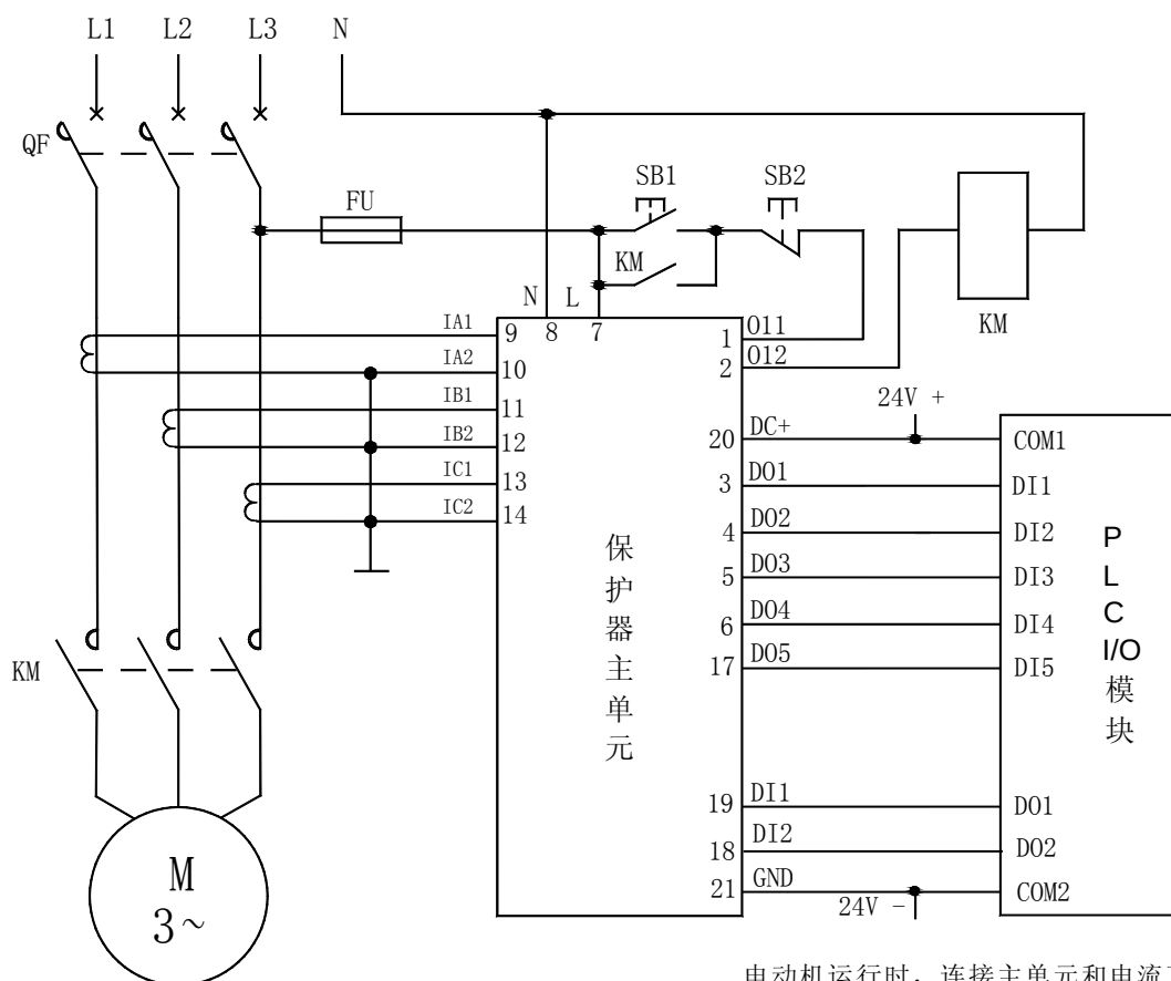
AMDPH-X/E621 系列电动机保护器 DO 连接 PLC 电气原理图
