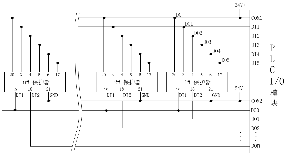
PLC 读取多台 AMDPH-X/E621 系列电动机保护器电气原理图
