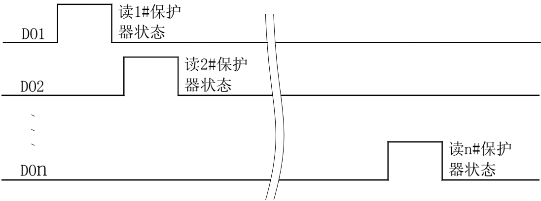
PLC 读取多台 AMDPH-X/E651 系列电动机保护器时序图
