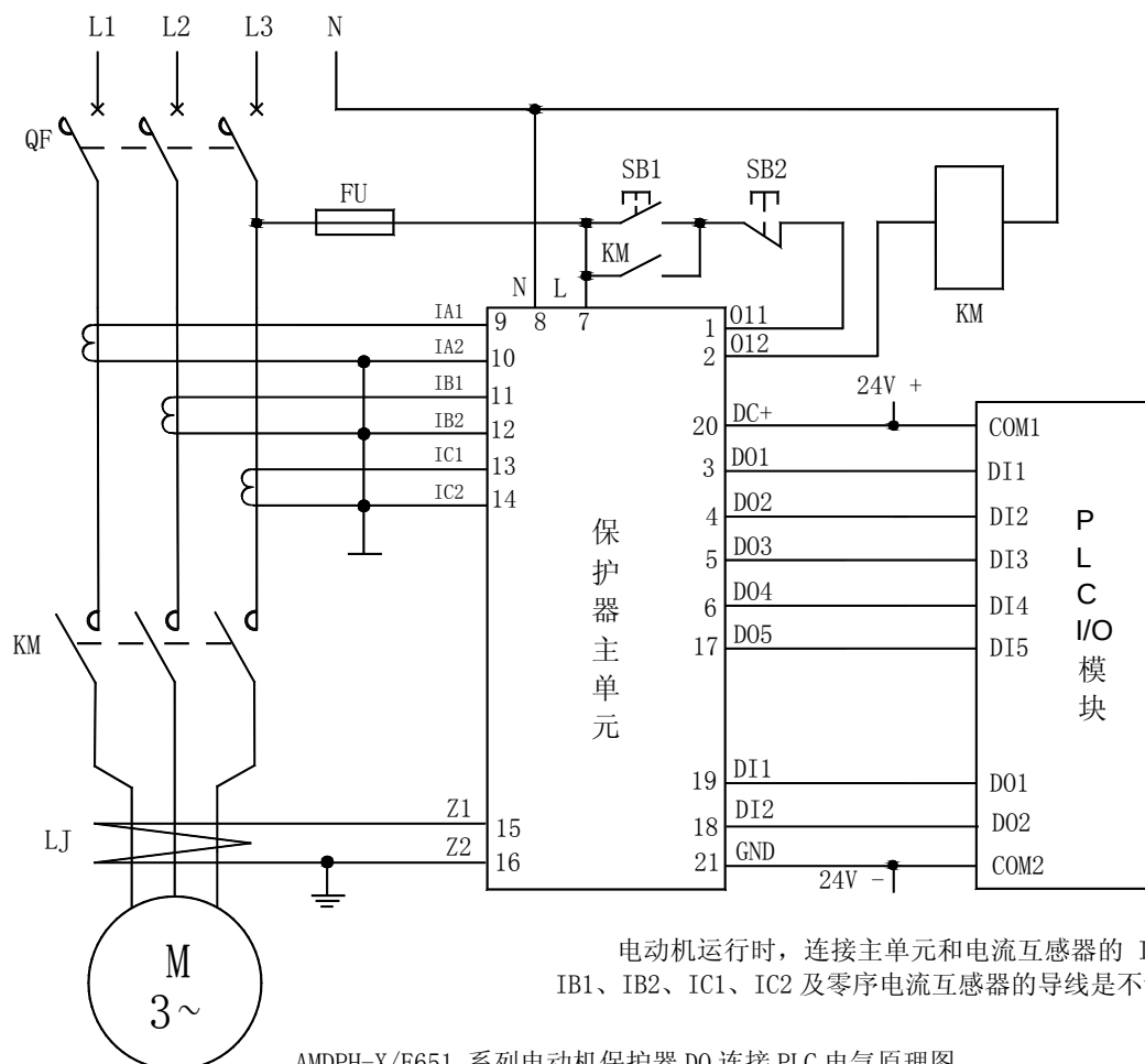
AMDPH-X/E651 系列电动机保护器 D0 连接 PLC 电气原理图
