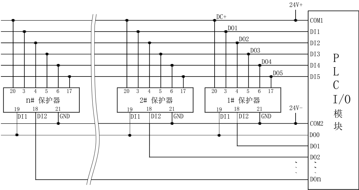
PLC 读取多台 AMDPH-X/E651 系列电动机保护器电气原理图
