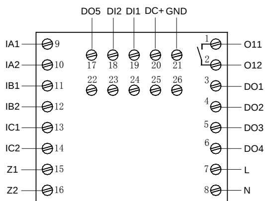
AMDPH-X/E651 系列保护器主单元接线端子图
