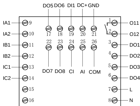
AMDPH-X/E701 系列保护器主单元接线端子图
