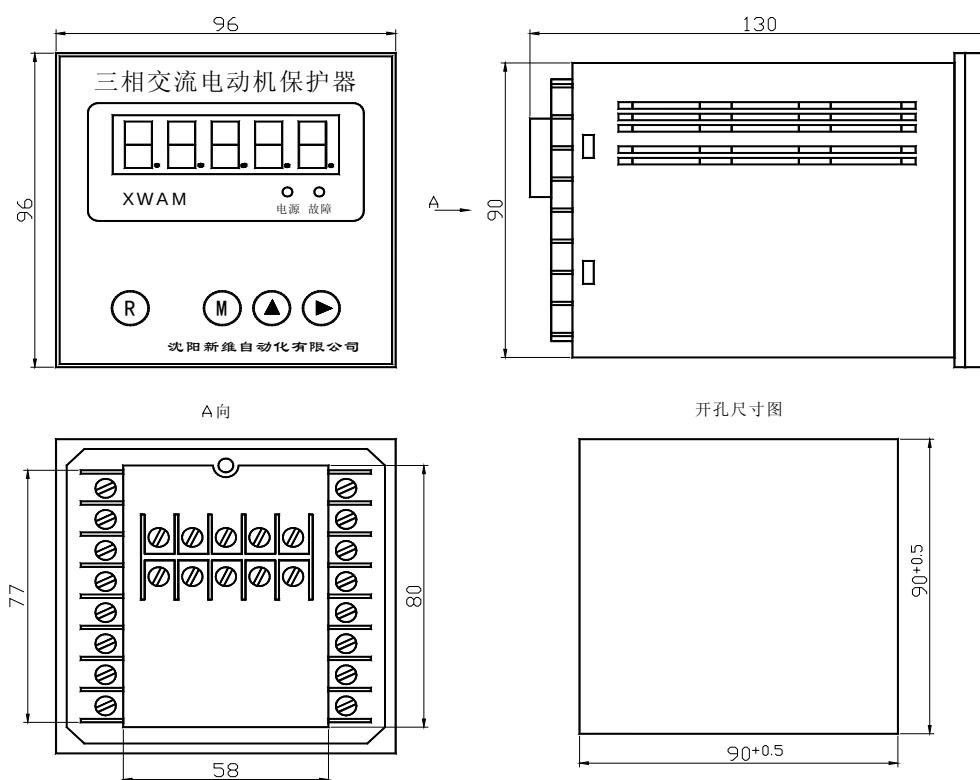
AMDPH-X/E701 系列电动机保护器主单元外形及安装孔尺寸
