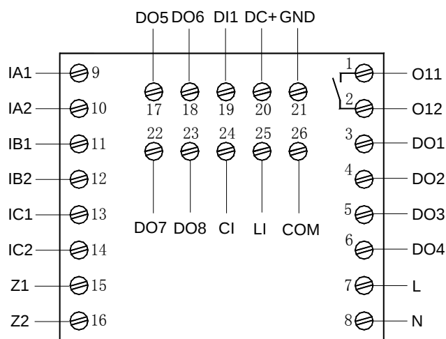
AMDPH-X/E711 系列保护器主单元接线端子图
