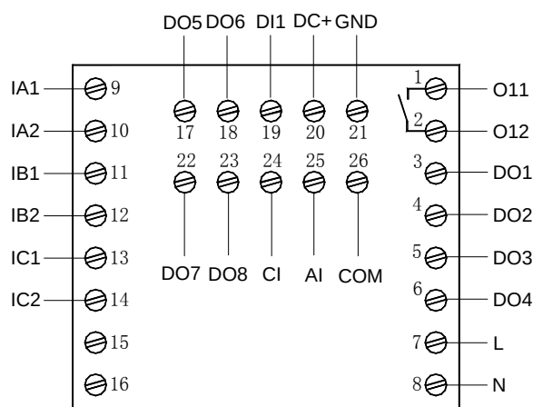
AMDPH-X/E721 系列保护器主单元接线端子图
