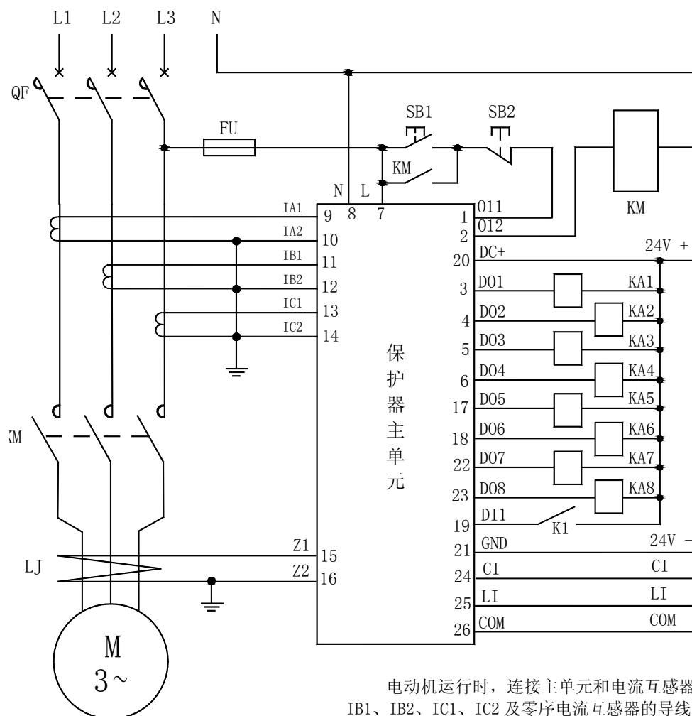
AMDPH-X/E751 系列电动机保护器 D0 连接继电器电气原理图
