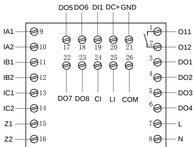
AMDPH-X/E751 系列保护器主单元接线端子图
