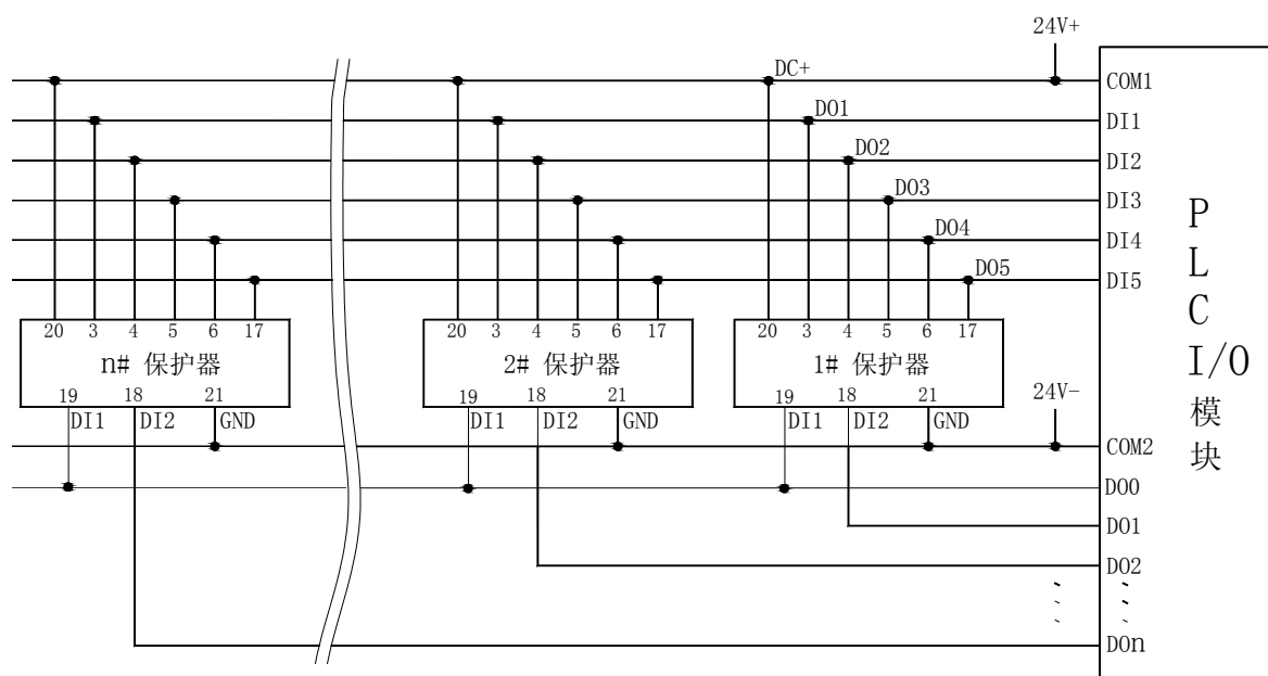
PLC 读取多台 AMDPH-X/E801 系列电动机保护器电气原理图
