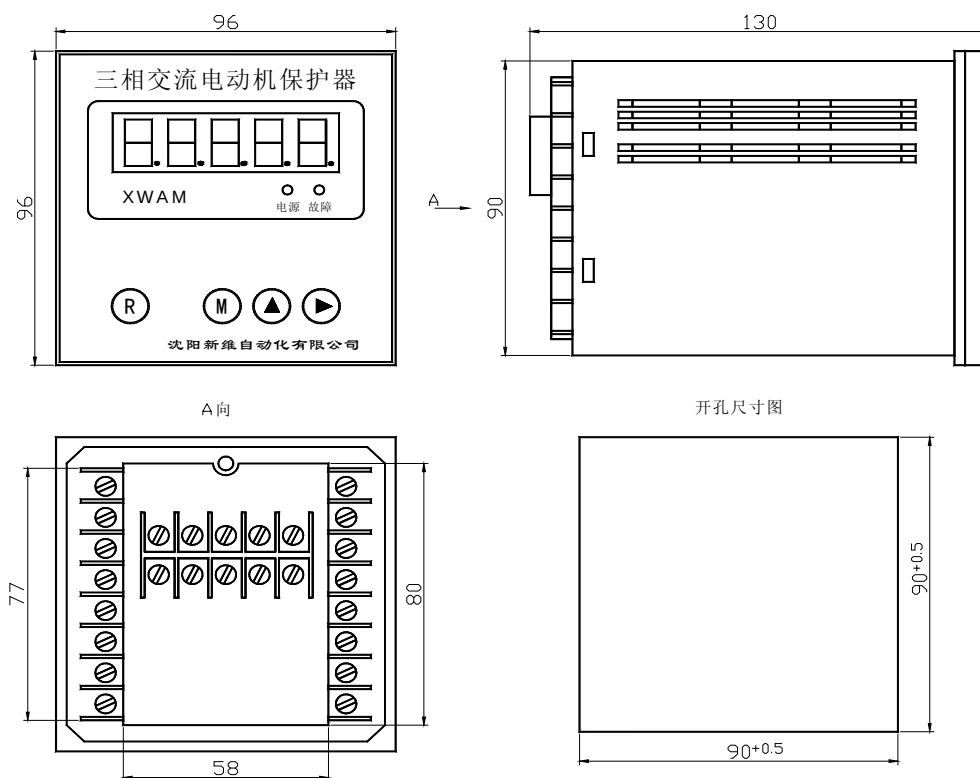
AMDPH-X/E801 系列电动机保护器主单元外形及安装孔尺寸
