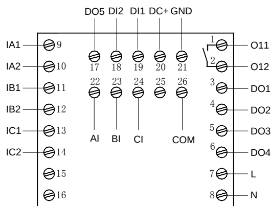
AMDPH-X/E801 系列保护器主单元接线端子图
