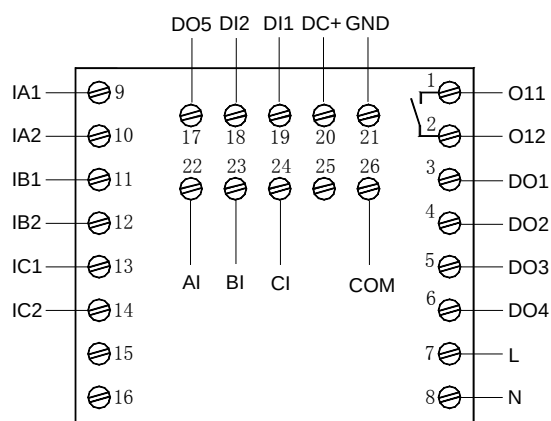
AMDPH-X/E821 系列保护器主单元接线端子图
