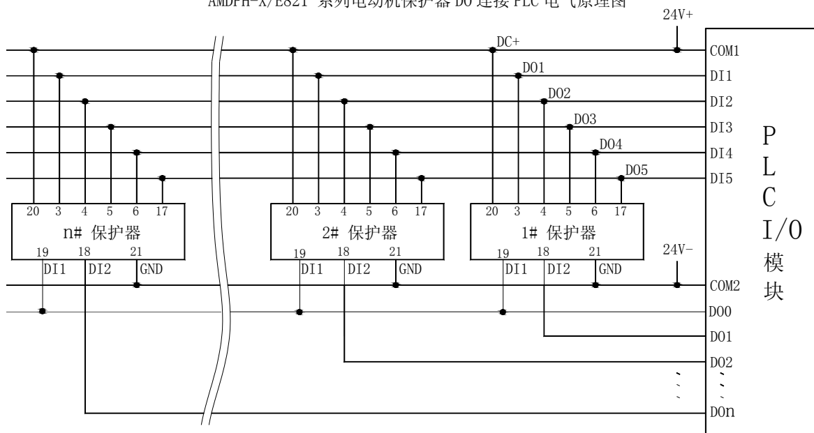
PLC 读取多台 AMDPH-X/E821 系列电动机保护器电气原理图
