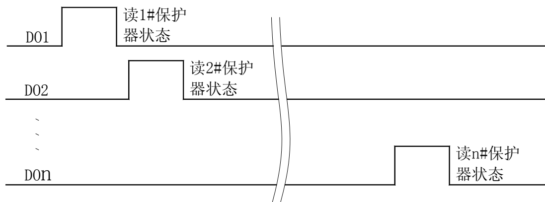
PLC 读取多台 AMDPH-X/E821 系列电动机保护器时序图
