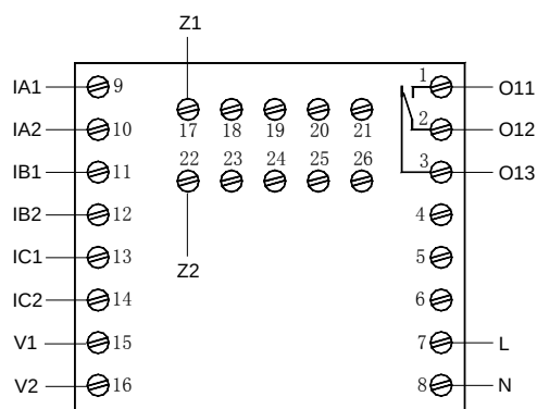
AMDPH-X/F061 系列保护器主单元接线端子图
