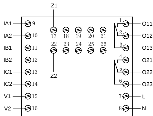
AMDPH-X/F062 系列保护器主单元接线端子图
