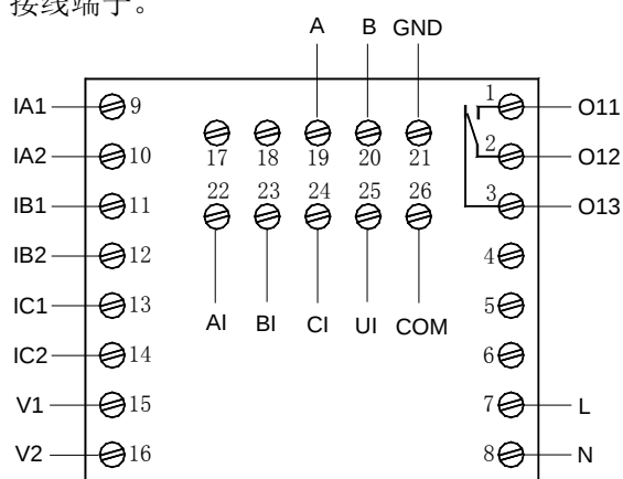
AMDPH-X/F441 系列保护器主单元接线端子图
