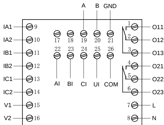
AMDPH-X/F442 系列保护器主单元接线端子图
