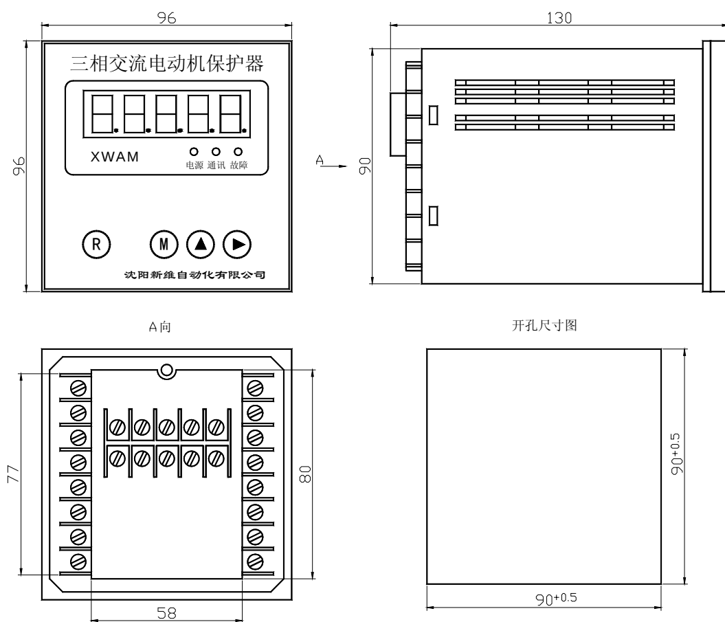
AMDPH-X/F44□ 系列电动机保护器主单元外形及安装孔尺寸
