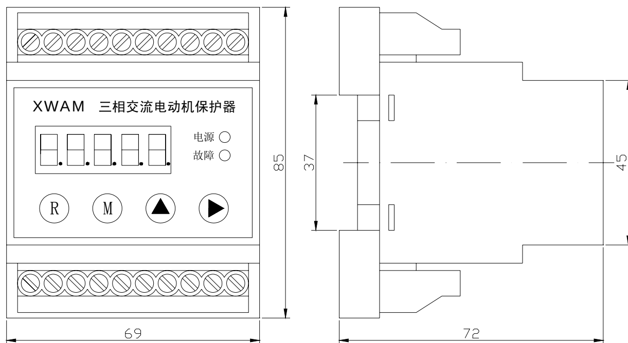
AMDS-□/DO5□ 系列电动机保护器主单元外形及安装孔尺寸
