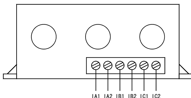
AMDS-□/D05□ 系列保护器电流检测单元接线端子图
