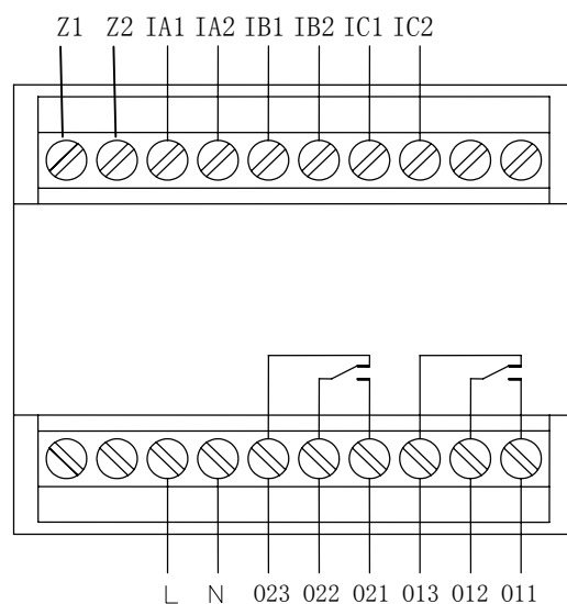
AMDS-□/D052 系列保护器主单元接线端子图
