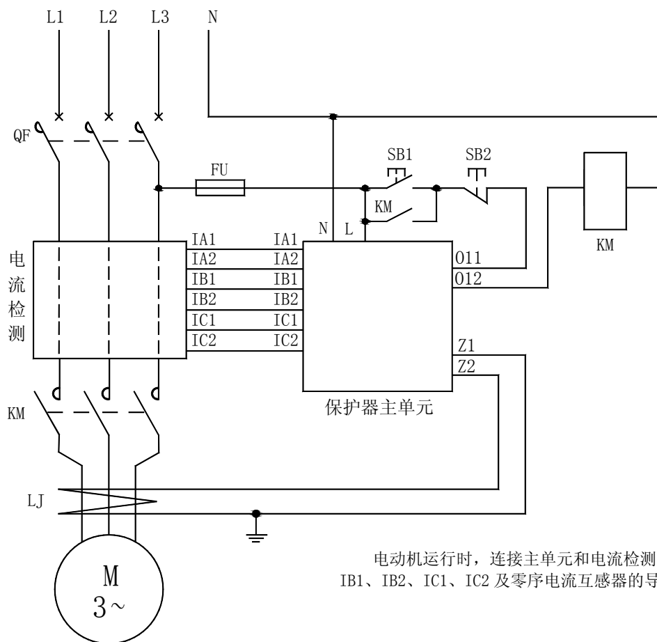
AMDS-□/D05□ 系列电动机保护器应用电气原理图
