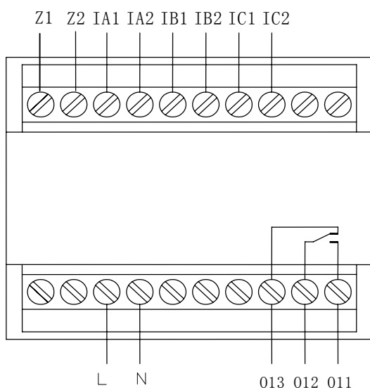
AMDS-□/D051 系列保护器主单元接线端子图 沈阳新维自动化有限公司
