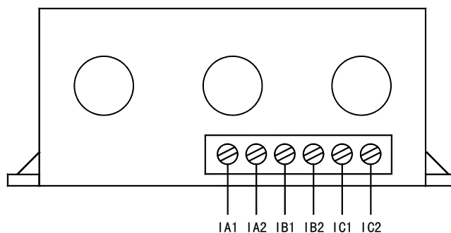
AMDS-□/D06□ 系列保护器电流检测单元接线端子图
