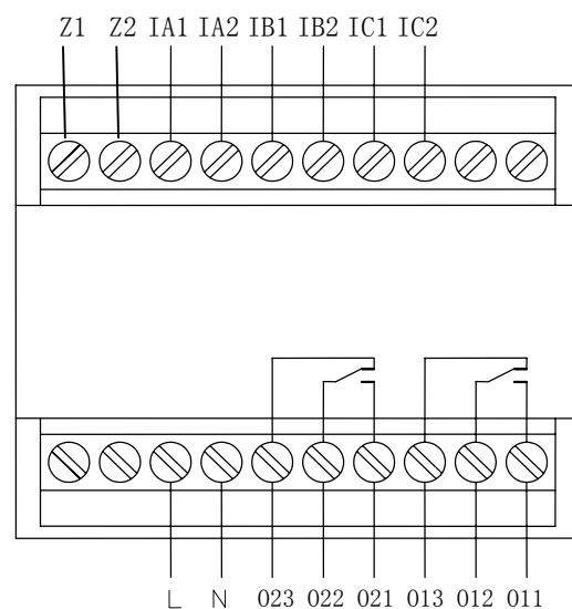
AMDS-□/D062 系列保护器主单元接线端子图
