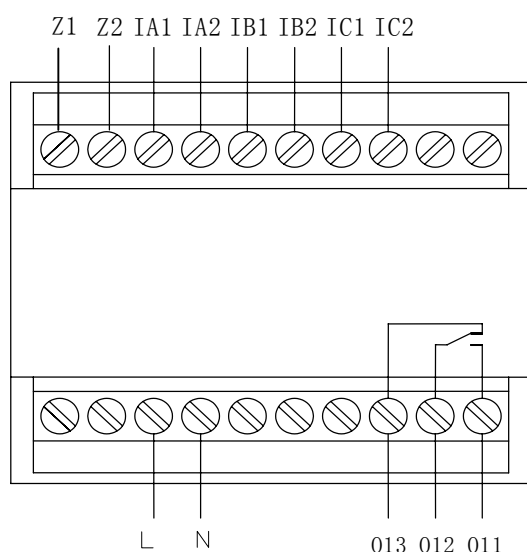
AMDS-□/D061 系列保护器主单元接线端子图 沈阳新维自动化有限公司
