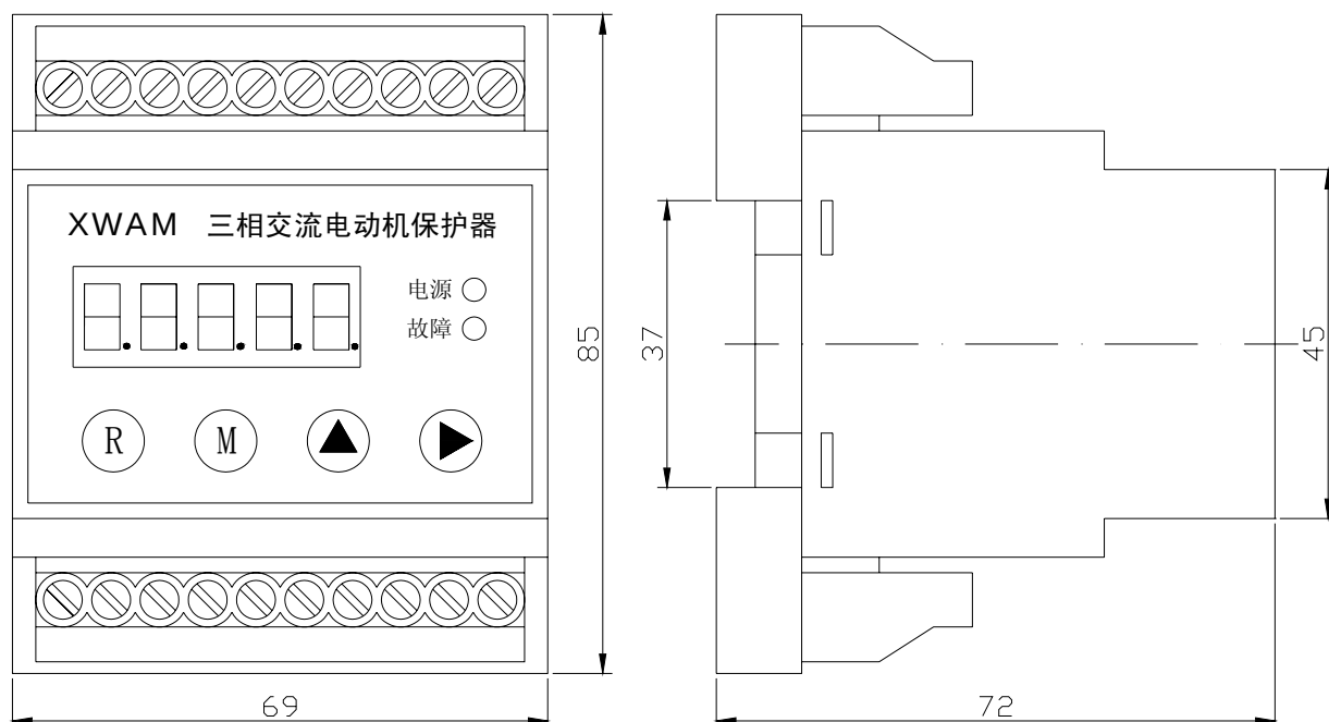
AMDS-□/D06□ 系列电动机保护器主单元外形及安装孔尺寸
