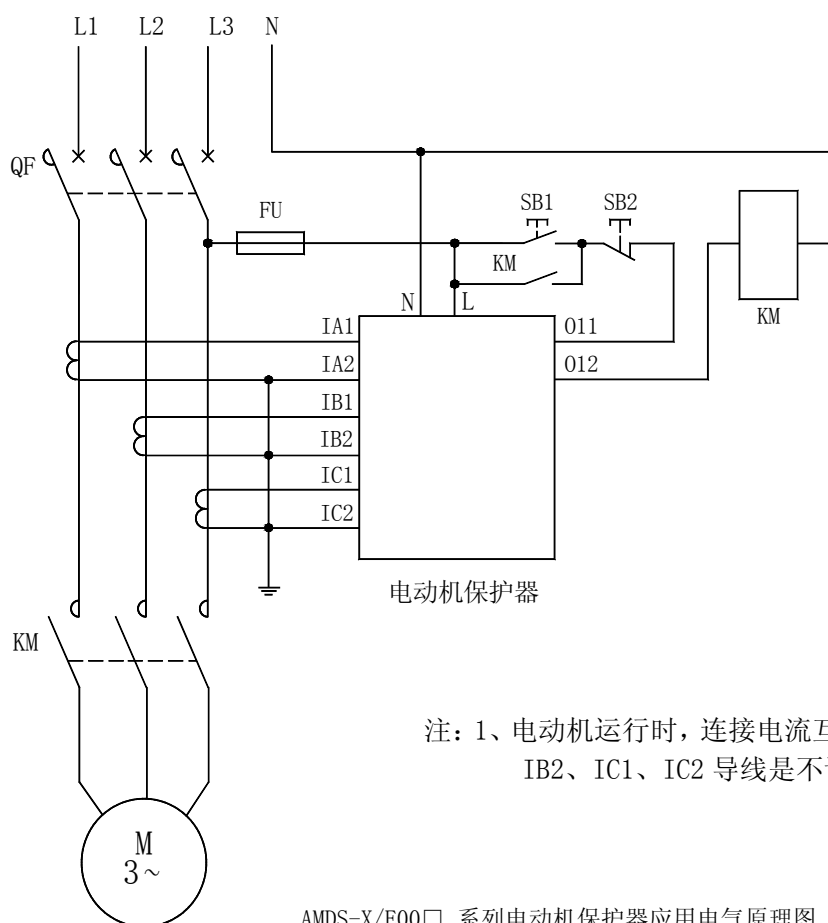
AMDS-X/E00□ 系列电动机保护器应用电气原理图
