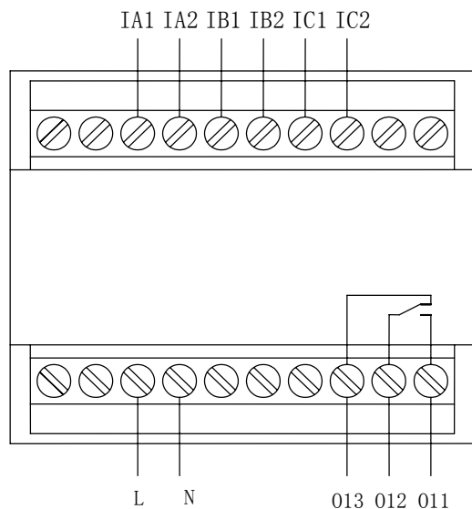
AMDS-X/E001 主单元端子图
