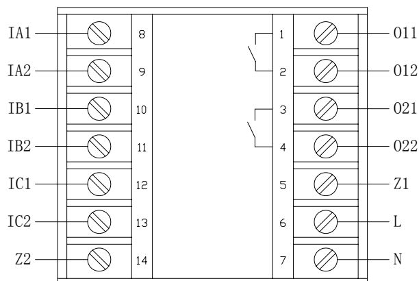
AMDTH-X/E053 主单元端子图
