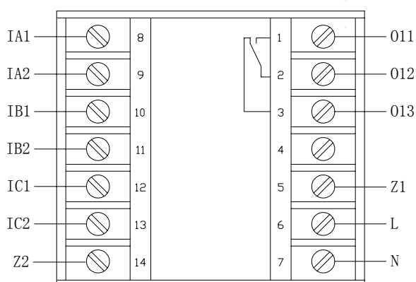
AMDTH-X/E051 主单元端子图
