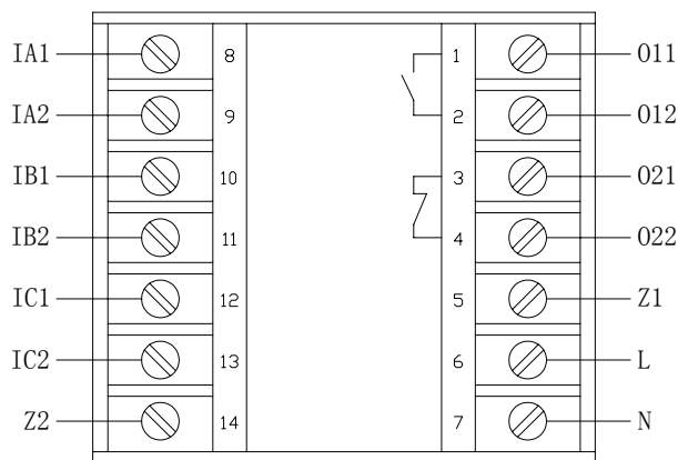
AMDTH-X/E054 主单元端子图
