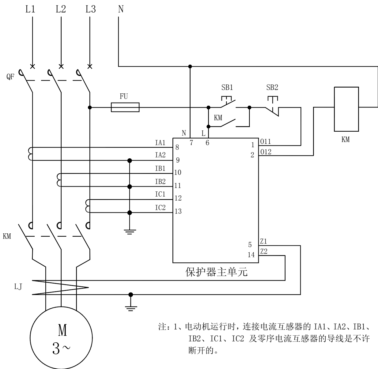
AMDTH-X/E054 系列电动机保护器应用电气原理图
