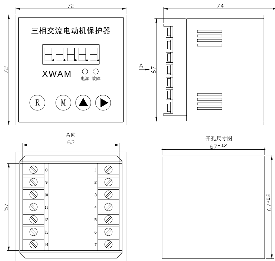
AMDTH-X/E05□ 系列电动机保护器主单元外形及安装孔尺寸
